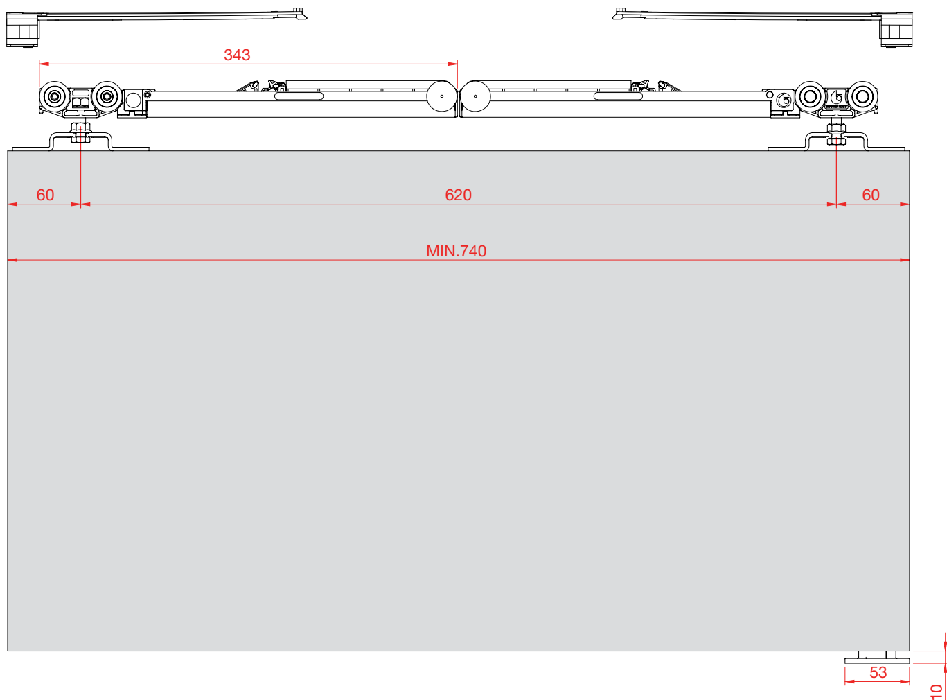
Montažni položaj za tekalno kolo Classic Fluid 70
