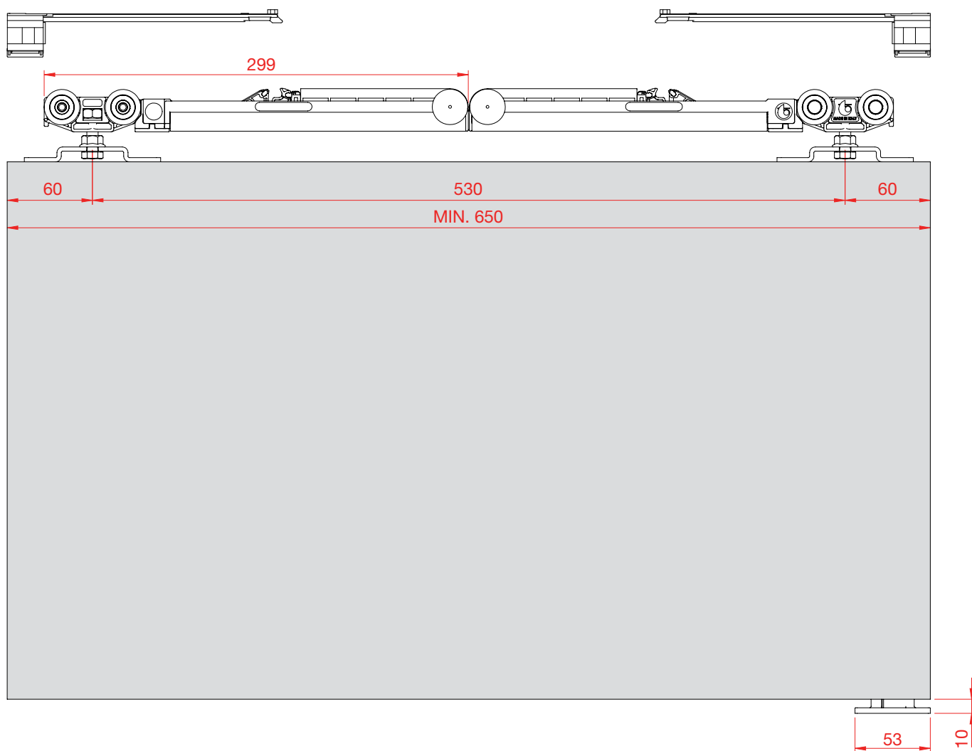
Montažni položaj za tekalno kolo Classic Fluid 50
