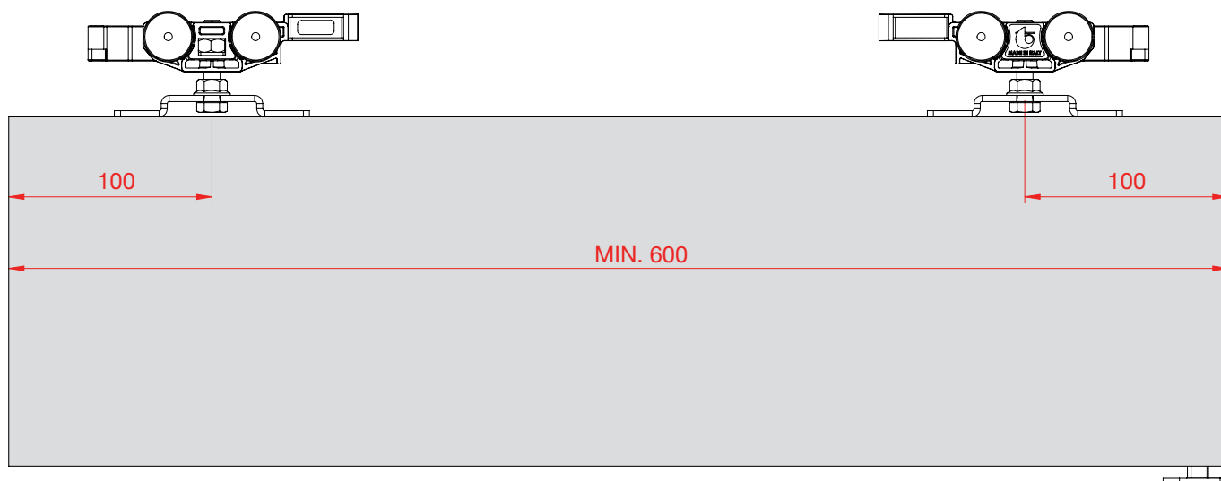
Montažni položaj tekalnega kolesa Classic Basic Standard
