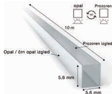
BLACK serija
