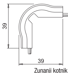
Zunanji kotnik
