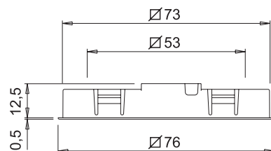
Hipso D-MOTION
