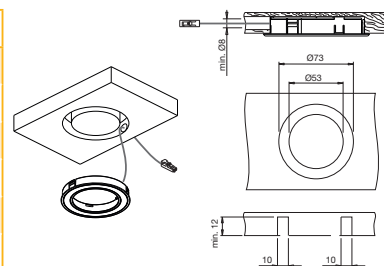
Odperta svetilka
