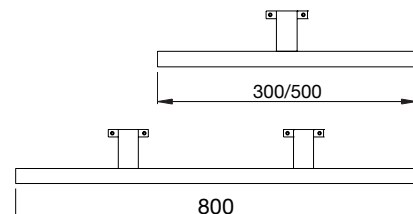
Podrobnost pritrditve
