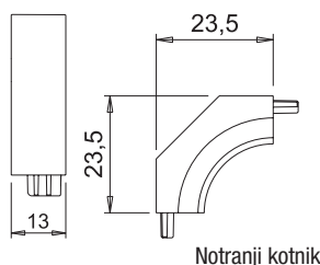
Notranji kotnik
