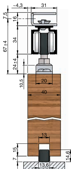
z nosilno prirobnico, pritrditveni kotnik stenske reže, stenska montaža
