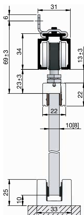
pritrditev s sponko, stenski pritrditveni kotnik
