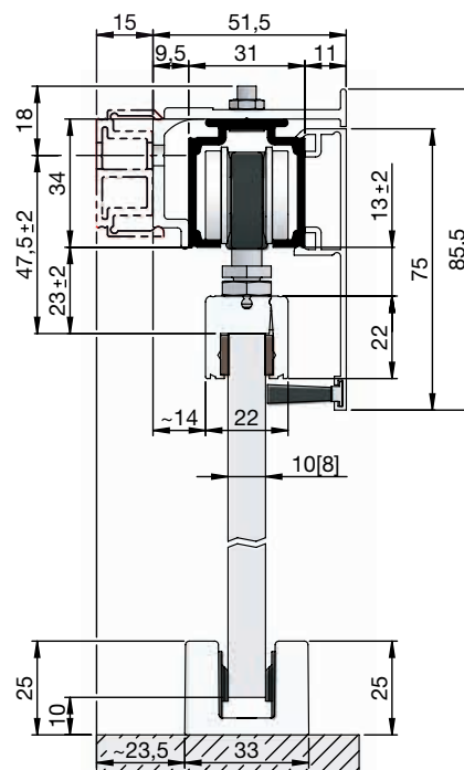
pritrditev s sponko, montažna tirnica, pokrivna letev H/G, enostranska s krtačo, distančni profil
