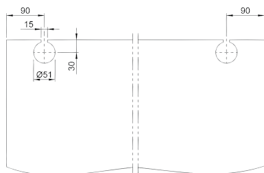
Okovje za steklo z zaustavljajčem
