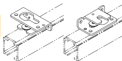
Pogled stropna montaža Pogled stenska montaža
