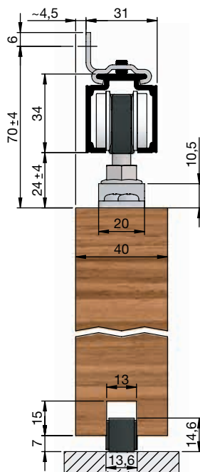
z nosilno prirobnico, stenski pritrditveni kotnik
