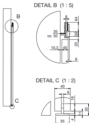
podrobnost lesena drsna vrata
