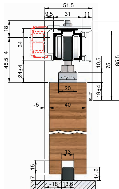
z nosilno prirobnico, montažna tirnica, pokrivna letev H/G, enostranska, distančni profil (rdeča)
