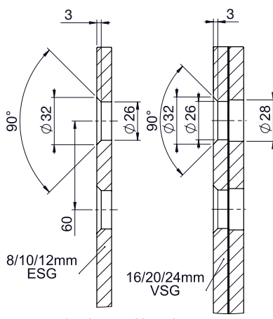
izvrtina v steklena drsna vrata
