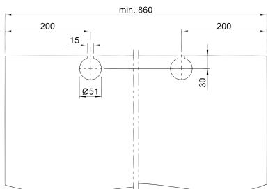
Okovje za steklo z blažilcem
