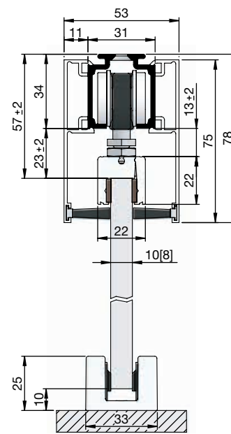
pritrditev s sponko, pokrivna letev H/G, obojestranska s krtačo
