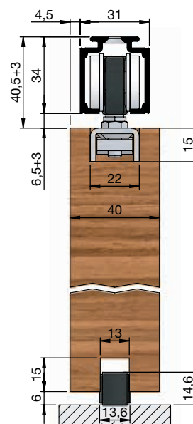
z jeklenim nosilnim profilom ME za minimalno vgradno višino
