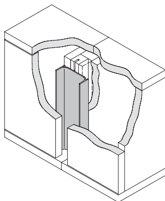
Profil pred stranskimi stenami
