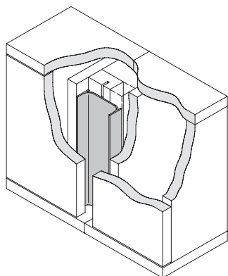
Profil med stranskimi stenami
