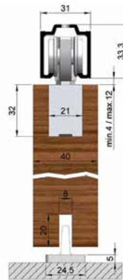
Z nosilnim profilom za minimalno vgradno višino, alu
