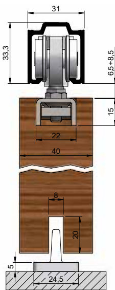
Z nosilnim profilom za minimalno vgradno višino, jeklo
