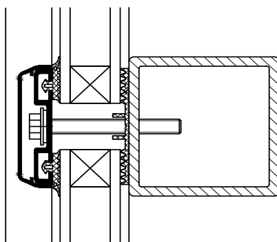
Rez A-A
