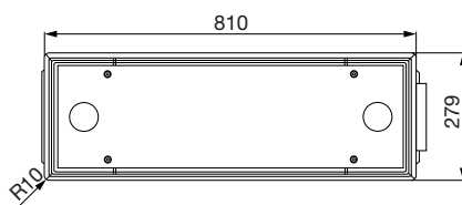
Različica B/notranje odvajanje zraka
