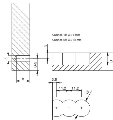
Skica izvrtin
