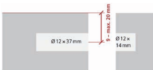
Mera izvrtine
